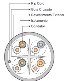
Cat6 Cu Data Cable
